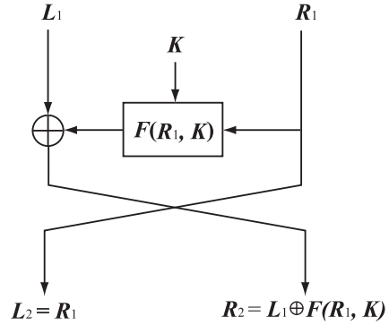
図5 Feistel型構造
